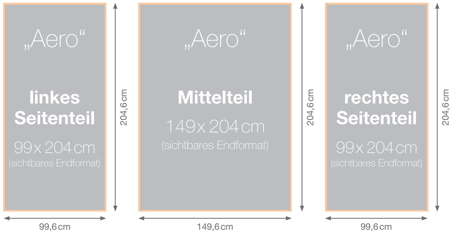
Messewand „Aero“ - Maße
